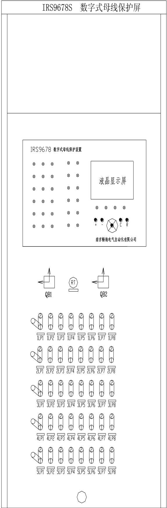
前视图
