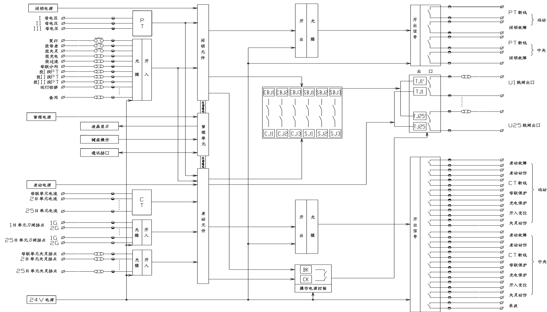
附图 1 保护原理图
