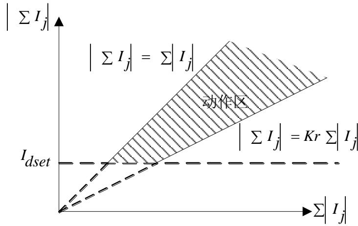
图 3-2 比率差动元件动作特性曲线
