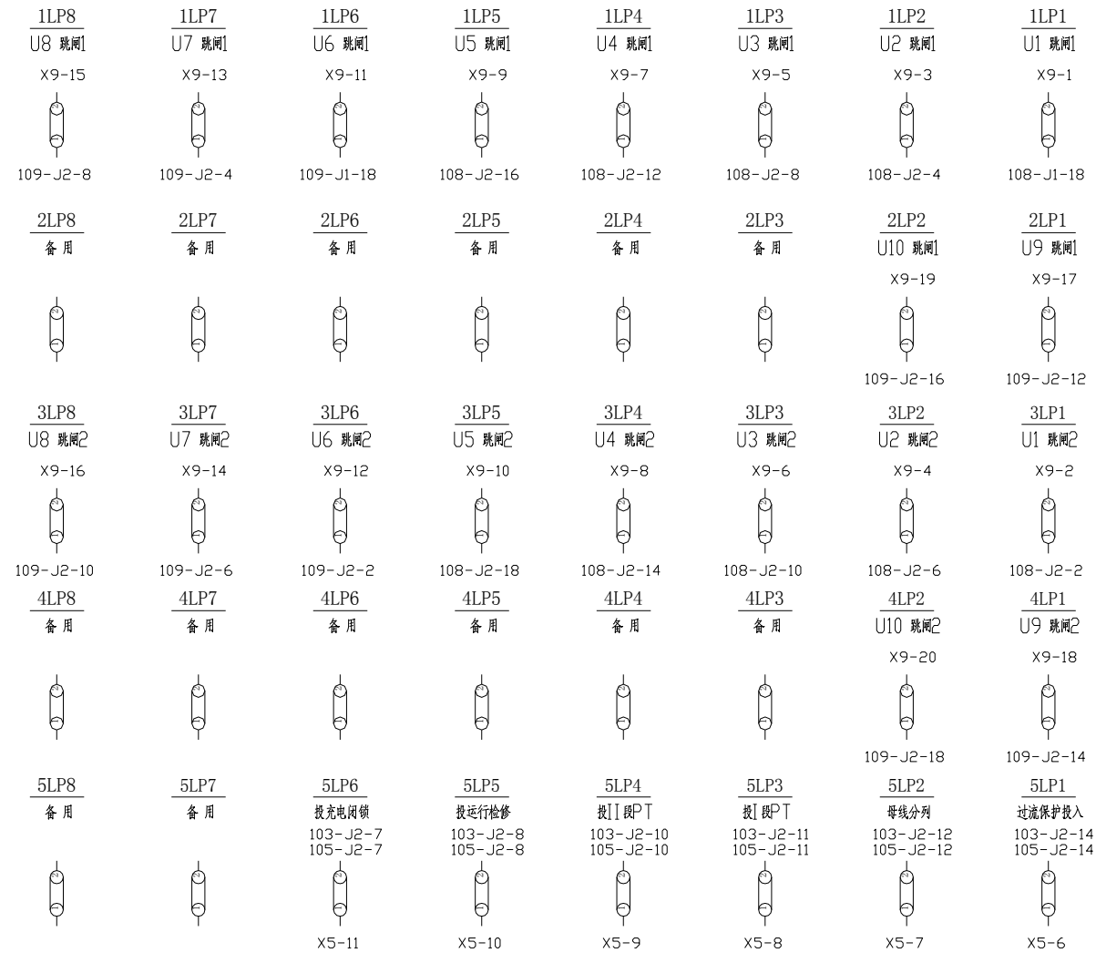
附图 9 IRS9678S 系列机柜压板接线图
