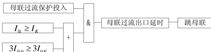
图 3-11 母联过流保护逻辑
