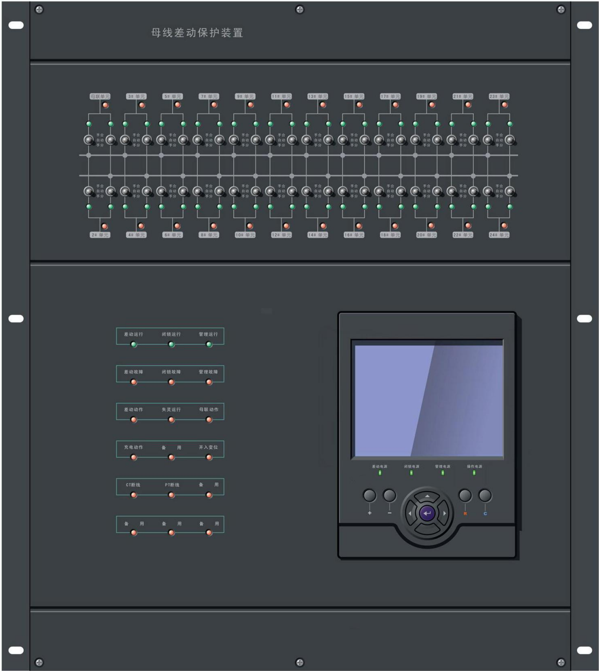
图 5-1 IRS9678A(B)面板布置图
