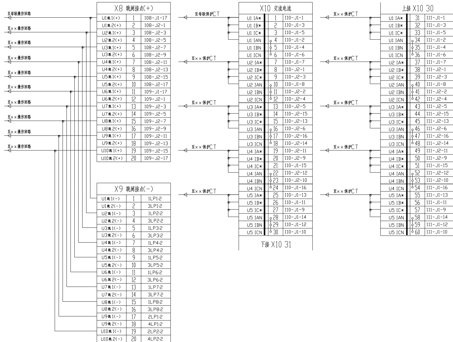
附图 7 IRS9678S 系列机柜右侧端子布置图
