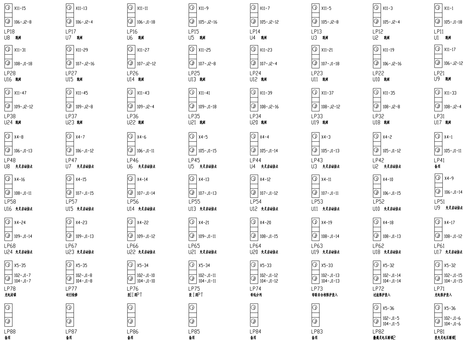
附图 5 IRS9678A(B)系列机柜压板接线图
